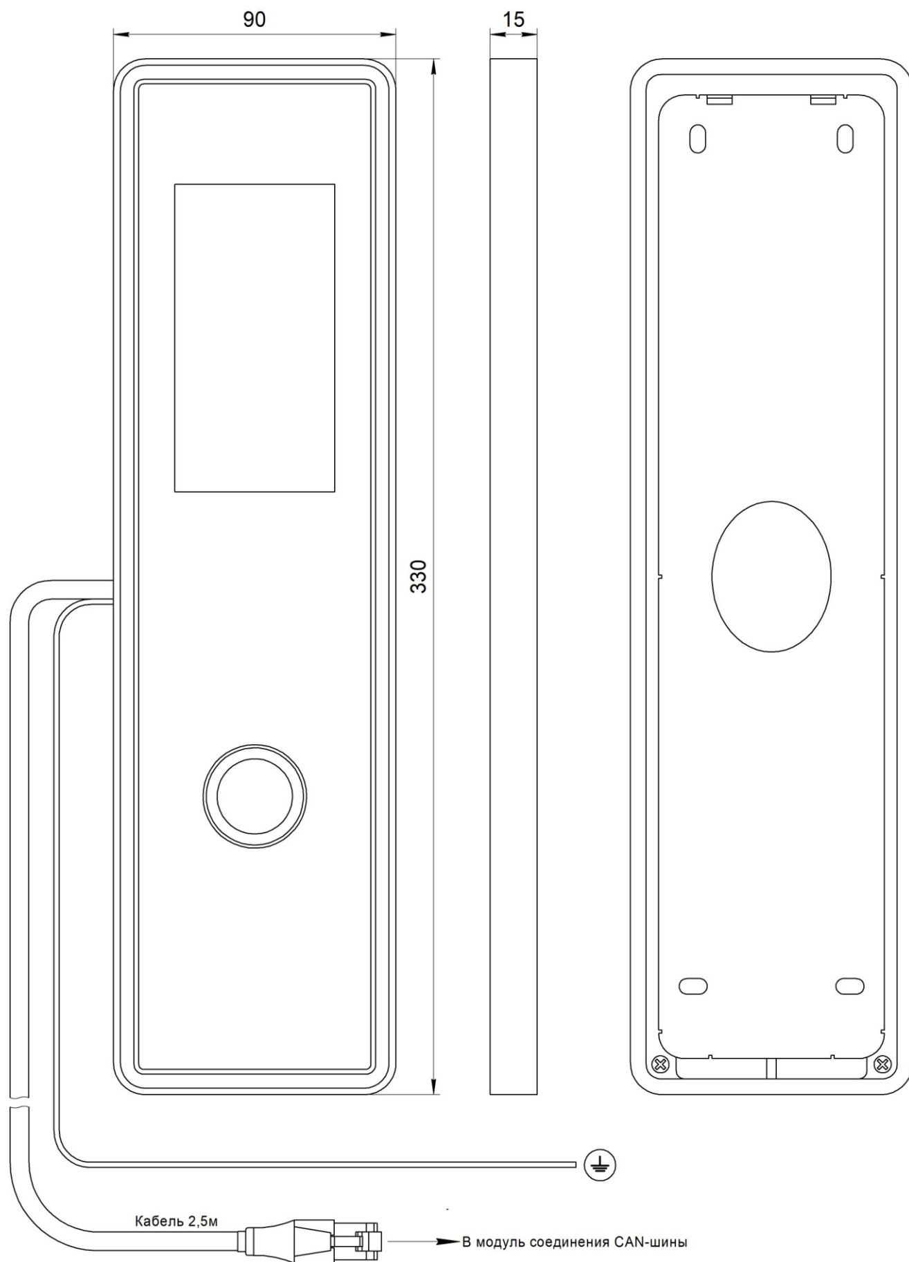
Рис.1 Внешний вид, габаритные и установочные размеры Вызывного поста ОБСИДИАН (жгут RJ45) НШЕК.468381.226
